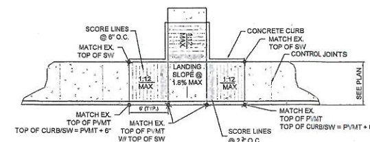
H/C RAMP DETAIL H.T.S.
